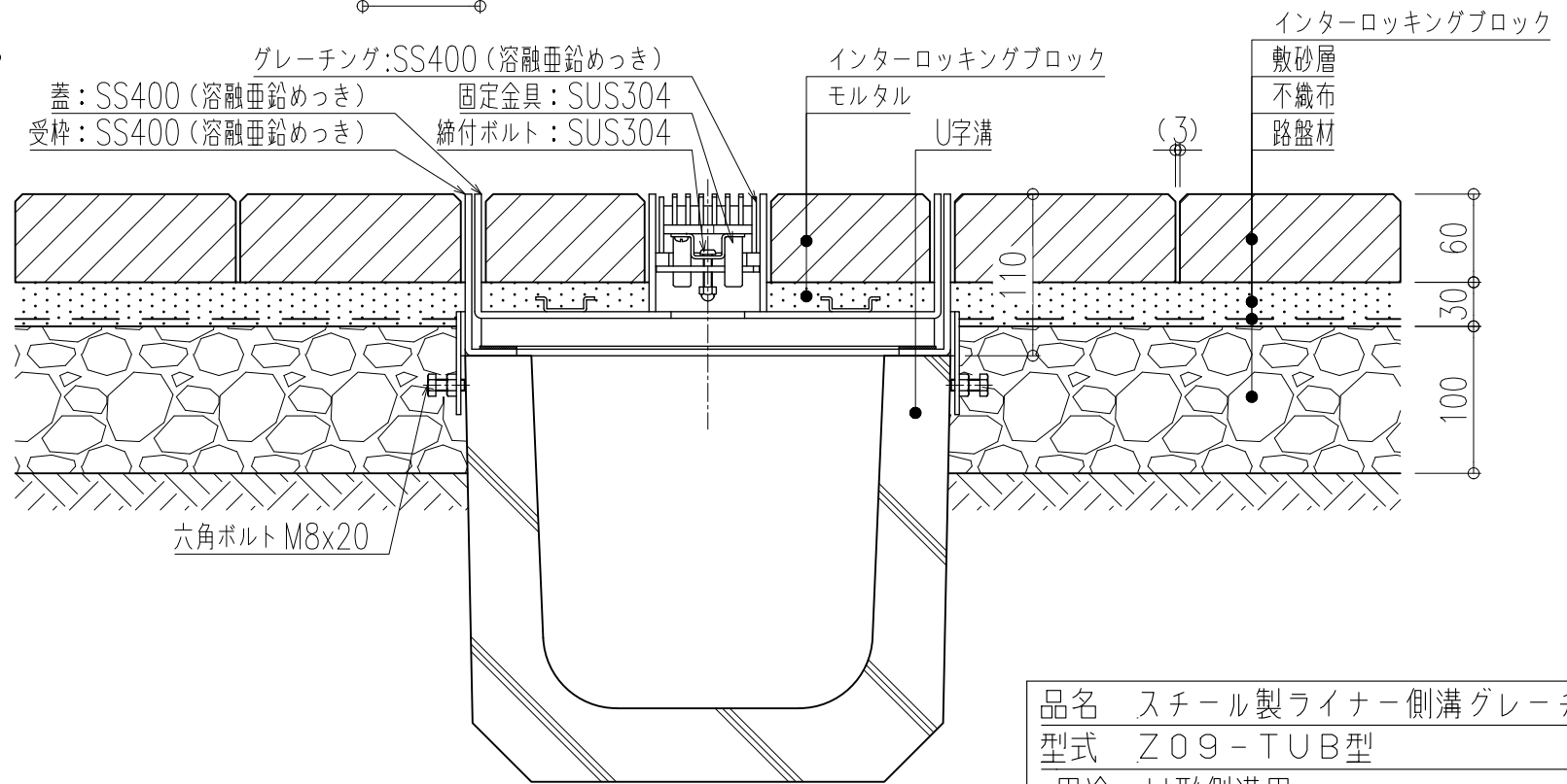
施工参考図
